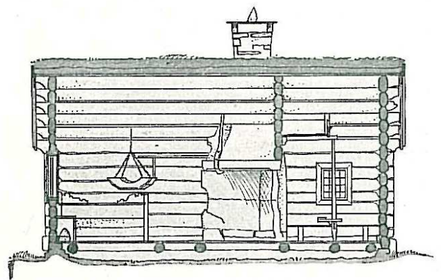
Stuen. Langsnitt. M. 1:100.
